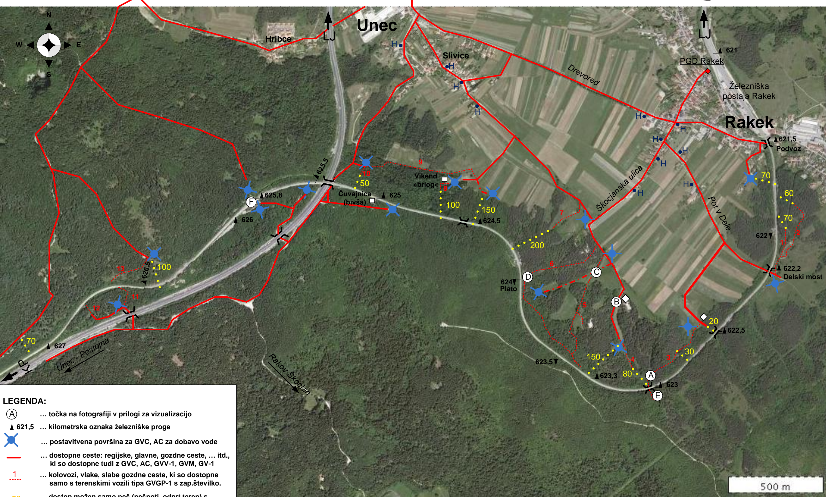
KARTA kilometrskih oznak in dostopov do železnice na odseku Rakek – meja občine Cerknica/Postojna, 621 – 627 km
